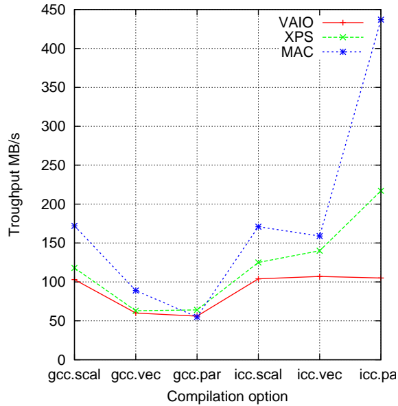
Figure 12. fdelay8.dsp benchmark
